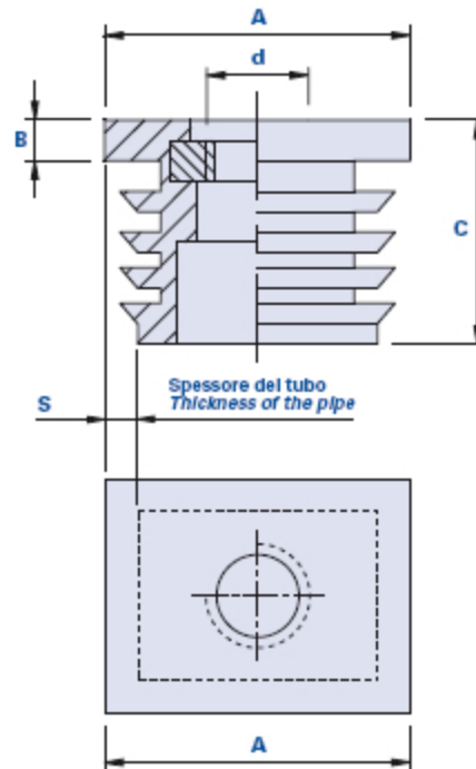
Abmessungen
